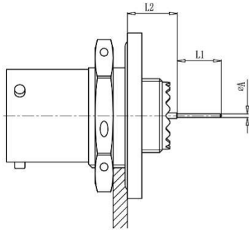
MS27496 receptacle
